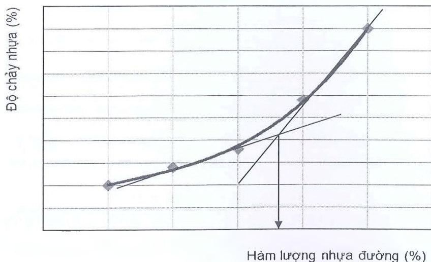
Hình A.2 – Biểu đồ quan hệ giữa hàm lượng nhựa và độ chảy nhựa (tham khảo)
