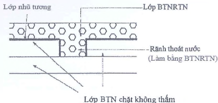
Hình G.13 – Rãnh thoát nước ngang bằng HHNRTN
