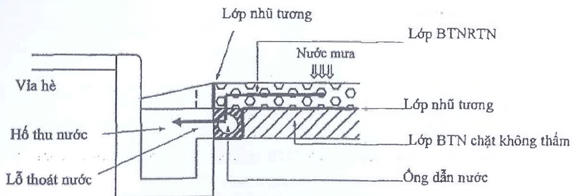
Hình G.8 – Rãnh thoát nước dạng chữ U (ví dụ 6)
