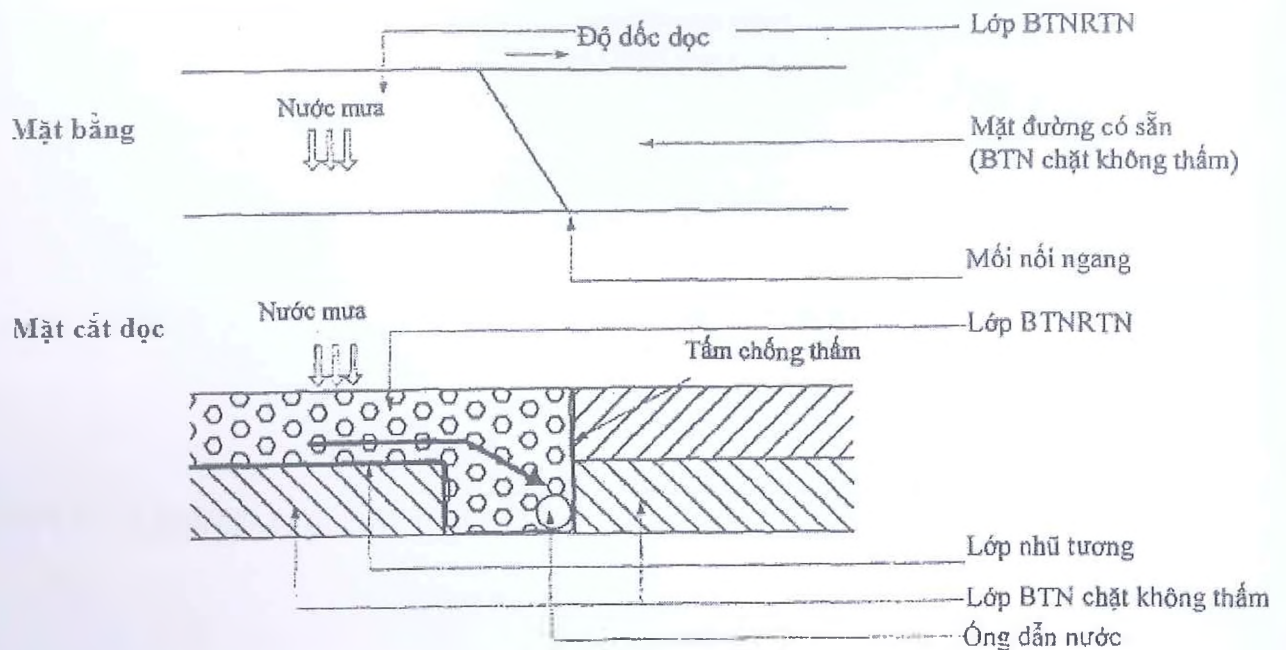
Hình G.12 – Rãnh bằng HHNRTN kết hợp ống dẫn nước dạng lưới hoặc xoắn
