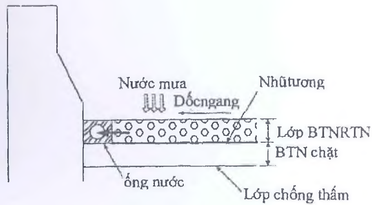
Hình G.17 – Đặt ống dẫn nước dạng lưới hoặc xoắn trong lớp HHNRTN
