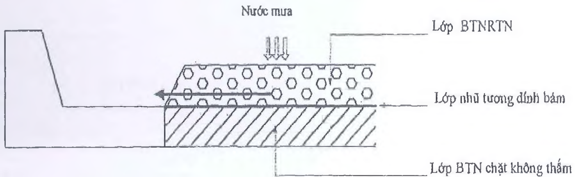
Hình G.1 – Rãnh thoát nước dạng chữ L (ví dụ 1)
