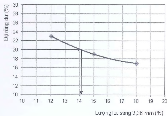
Hình A.1 – Biểu đồ quan hệ giữa lượng lọt sàng 2,36 mm và độ rỗng dư
